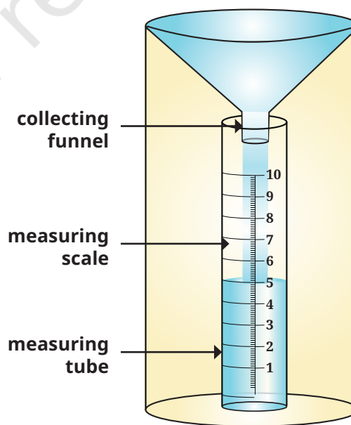
Fig. 2.6. Rain gauge
